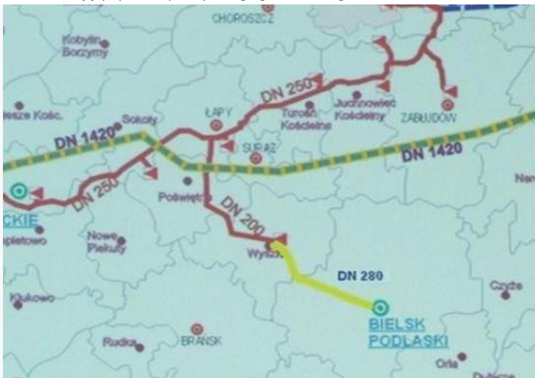
Rys. 3. Stan istniejący systemu przesyłowego gazu ziemnego
