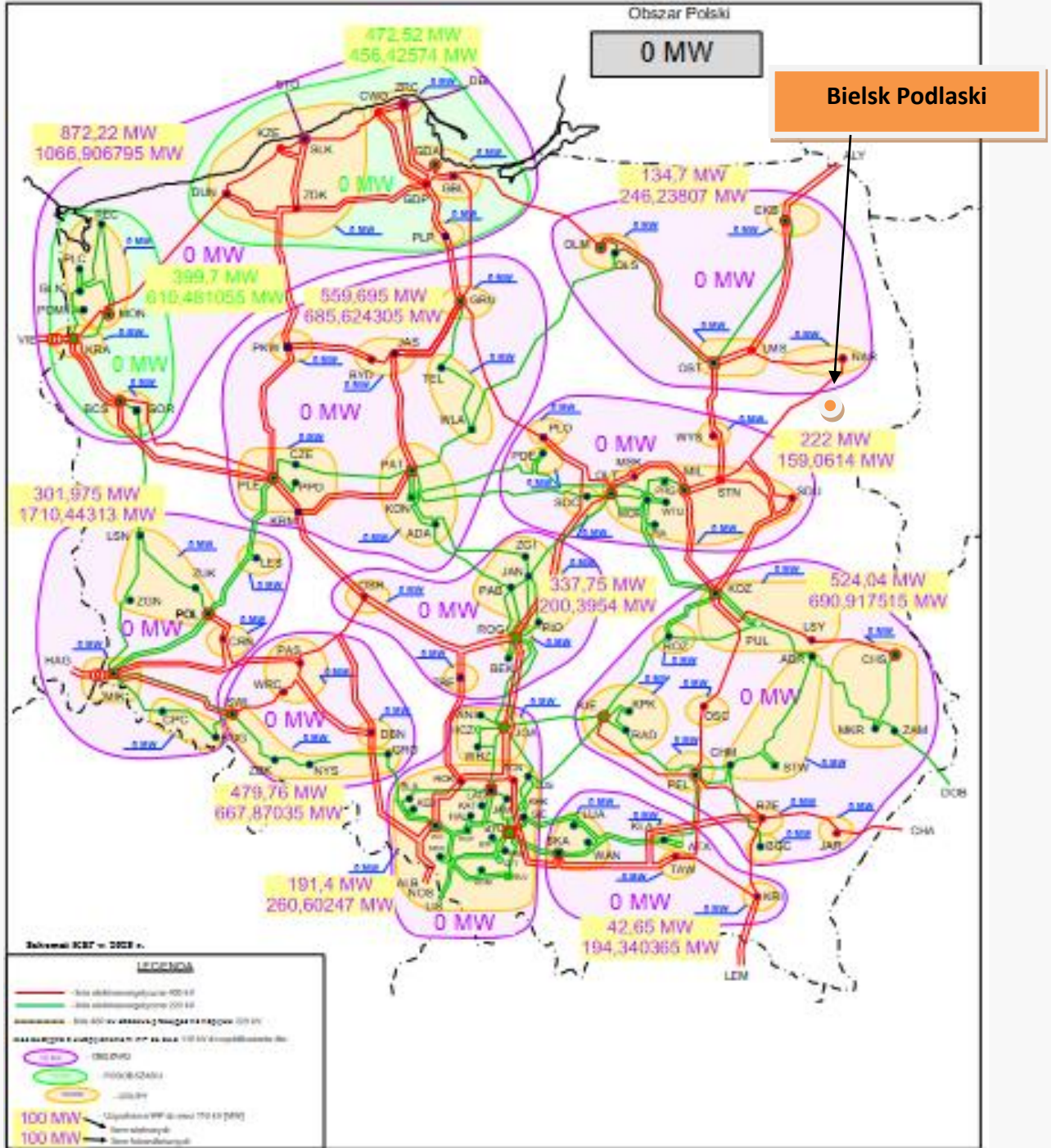
Rys.6. Schemat sieci przesyłowej z dostępnymi mocami przyłączeniowymi – planowana rozbudowa na rok 2028
